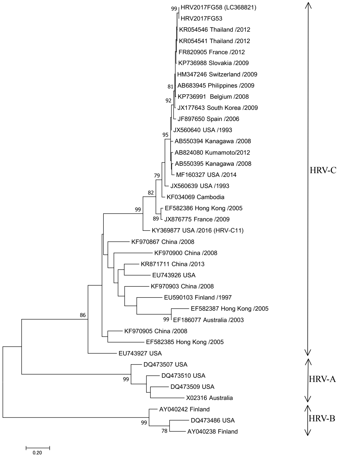
図 2. 本事例から検出されたライノウイルスの分子系統樹 (ML 法) 5' -UTR-VP4/VP2 領域 (441bp) を用いた系統樹解析 HRV2017FG53 および HRV2017FG58 は本事例から検出された株 (Accession No. LC368821)
