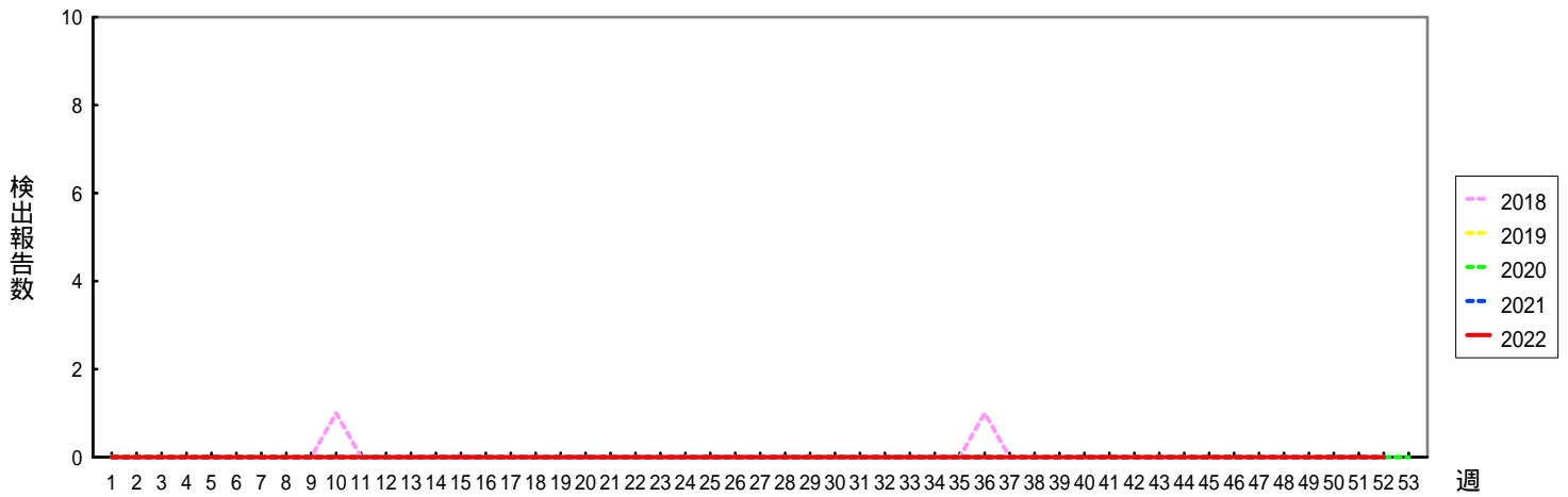
01&0139以外のV.cholerae
