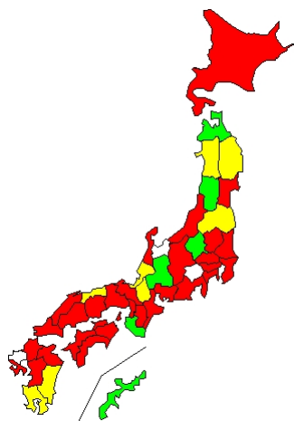
893 例 Coxsackievirus A6
