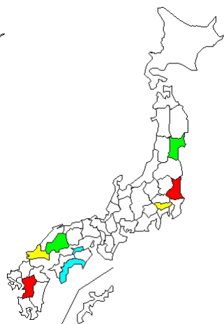
58 例 Enterovirus NT
