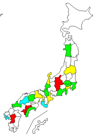
112 例 Rhinovirus
