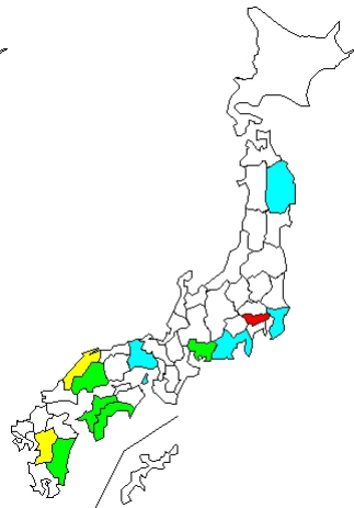
51 例 Coxsackievirus A6
