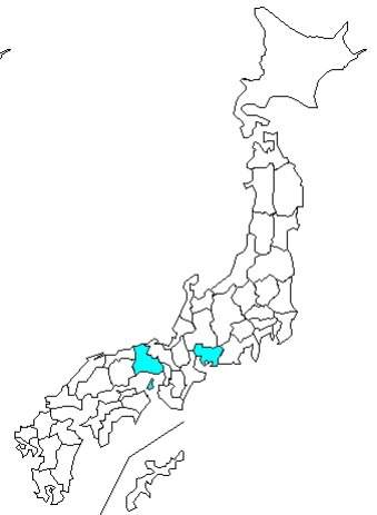
2 例 Echovirus 9
