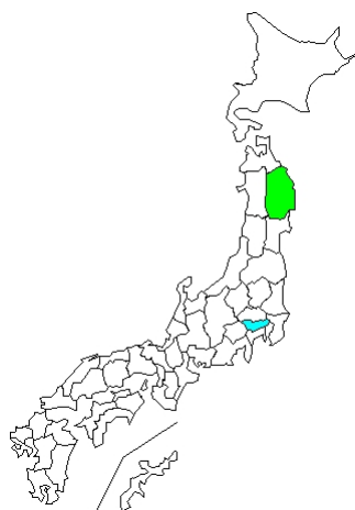
3 例 B19 virus
