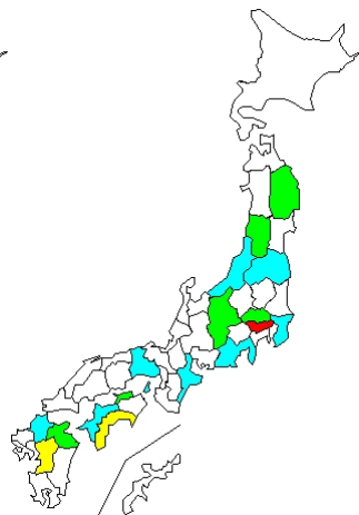
54 例 Rhinovirus
