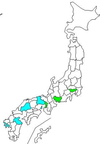
13 例 Coxsackievirus A9
