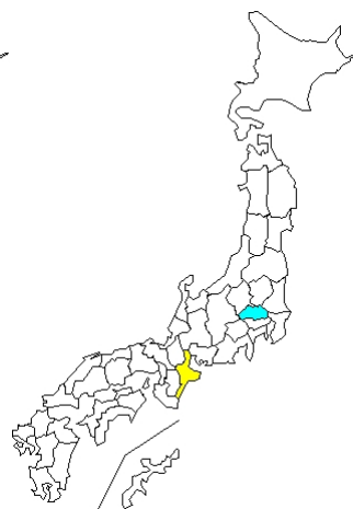
8 例 HCoV NT
