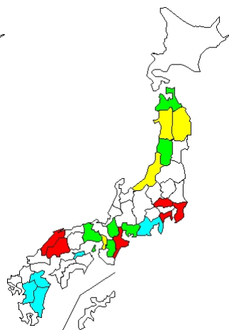
195 例 Human metapneumovirus
