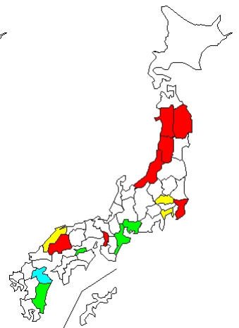
134 例 Parainfluenza virus 3
