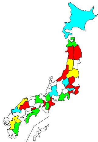
357 例 Rhinovirus
