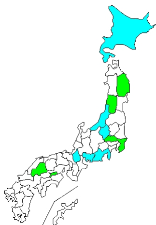
21 例 Adenovirus 2
