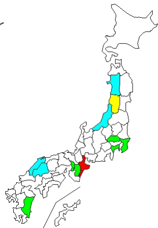
48 例 Parainfluenza virus 1
