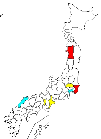
57 例 Human bocavirus
