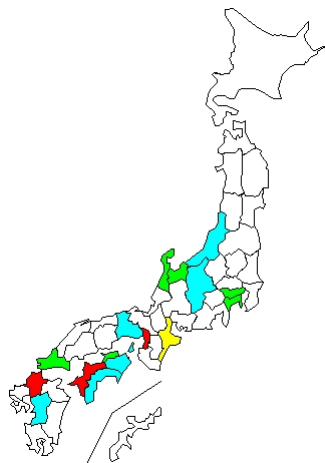
74 例 Coxsackievirus A6
