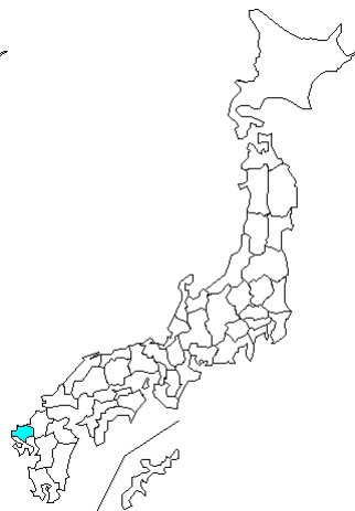
1 例 Enterovirus 71
