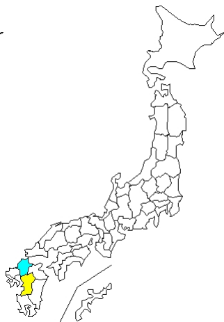
9 例 Coxsackievirus A16
