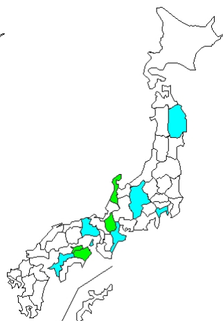
16 例 Rhinovirus
