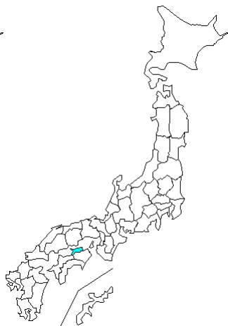
1 例 Coxsackievirus A10
